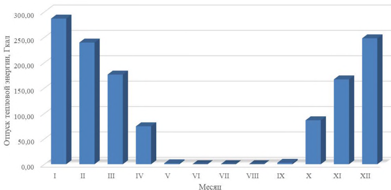
Рисунок 1.3 – Оптимальный температурный график отпуска тепловой энергии для котельной с. Боголюбовка
